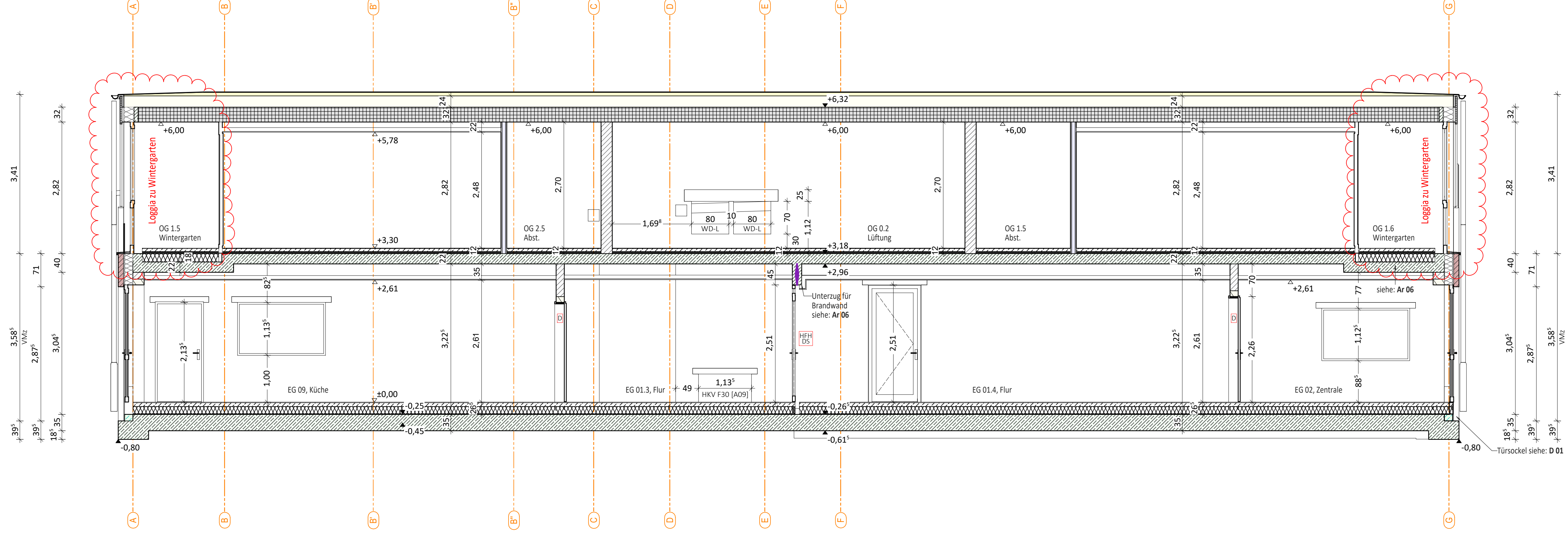
Schnitt B Küche - Flur - Zentrale - Wohnungen und Lüftungen im 1.OG
