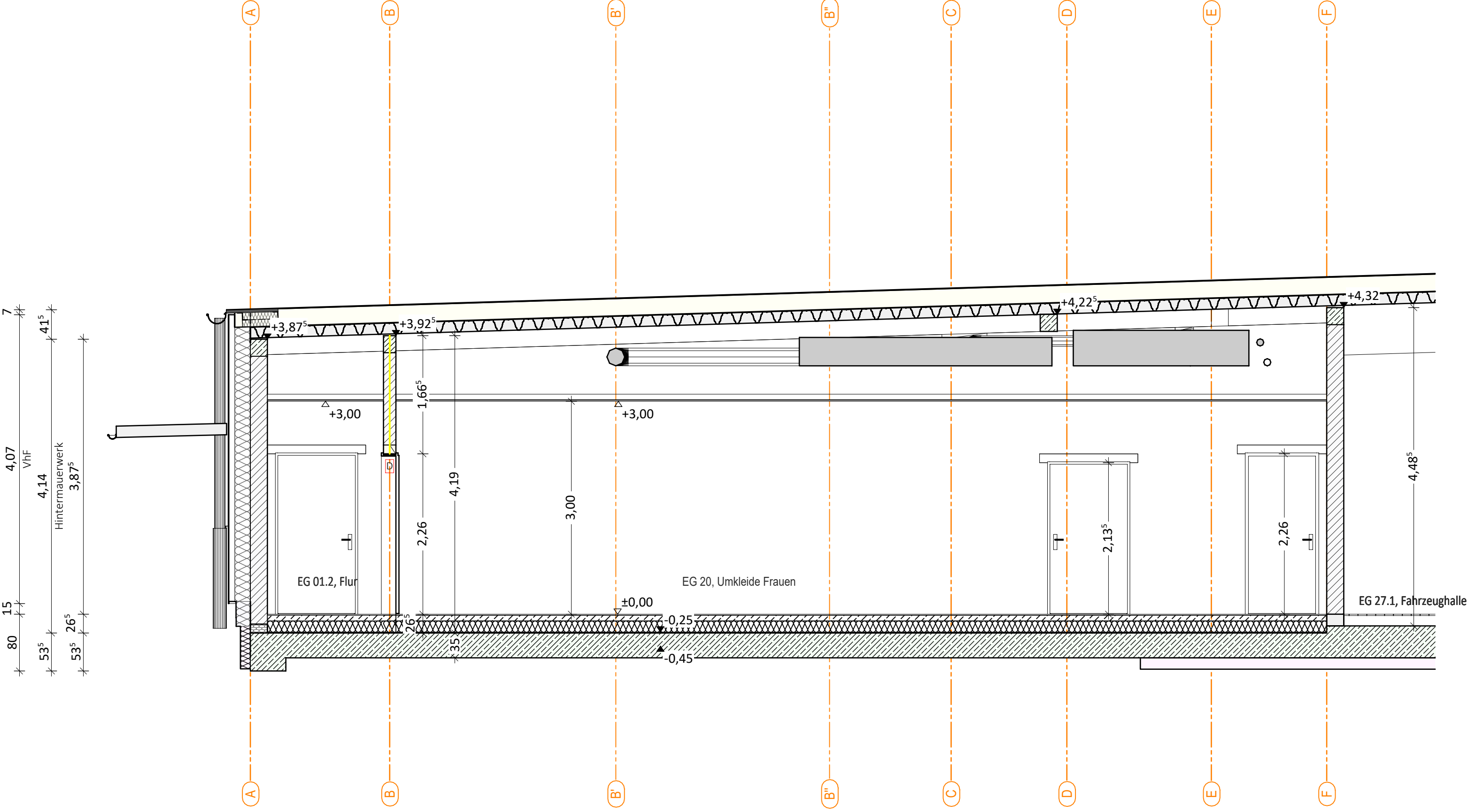
Schnitt G Flur - Umkleide D. mit Durchgang zur Fahrzeughalle
