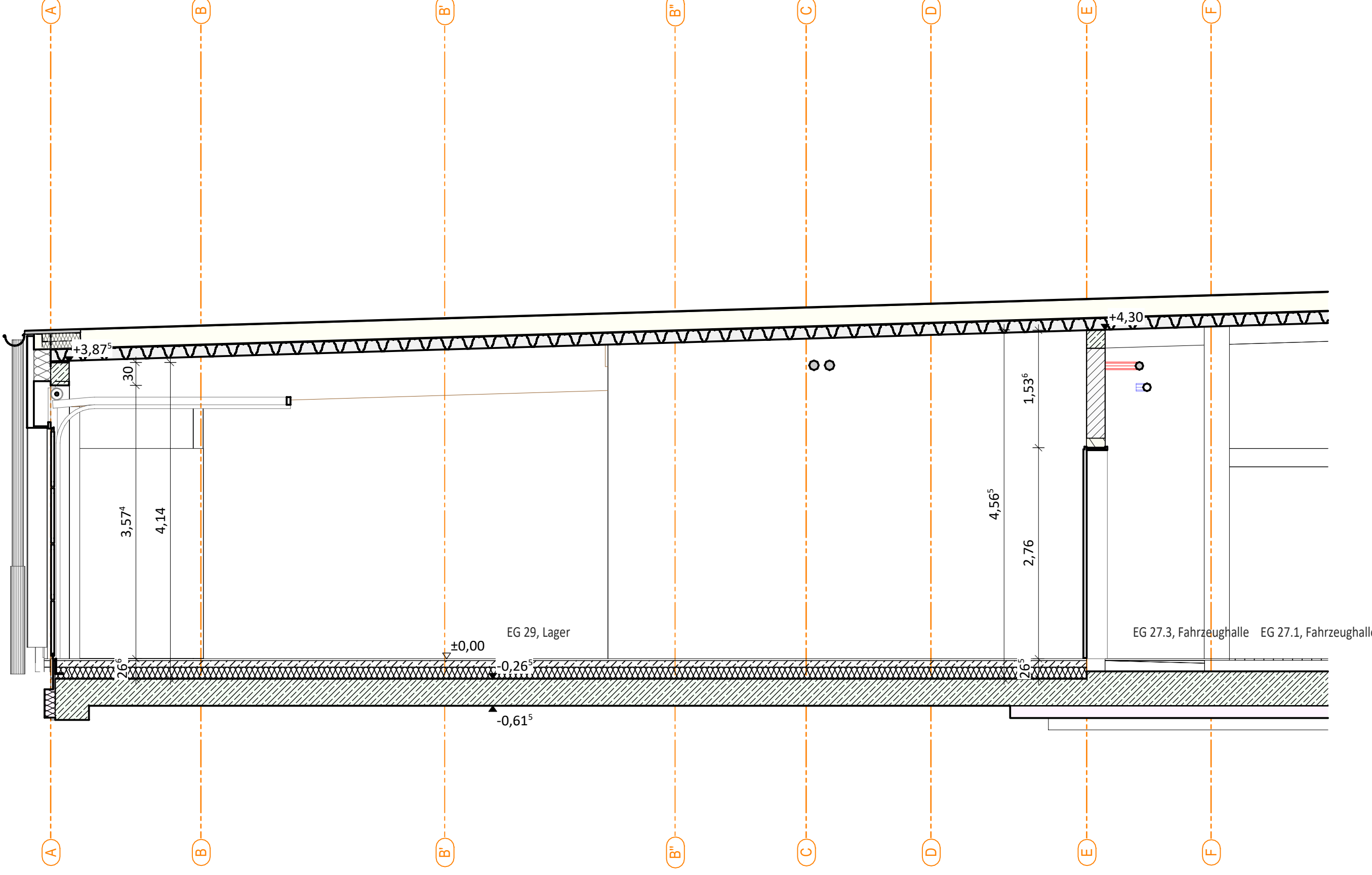
Schnitt H Lager mit eingestelltem Tauschraum - Fahrzeughalle
