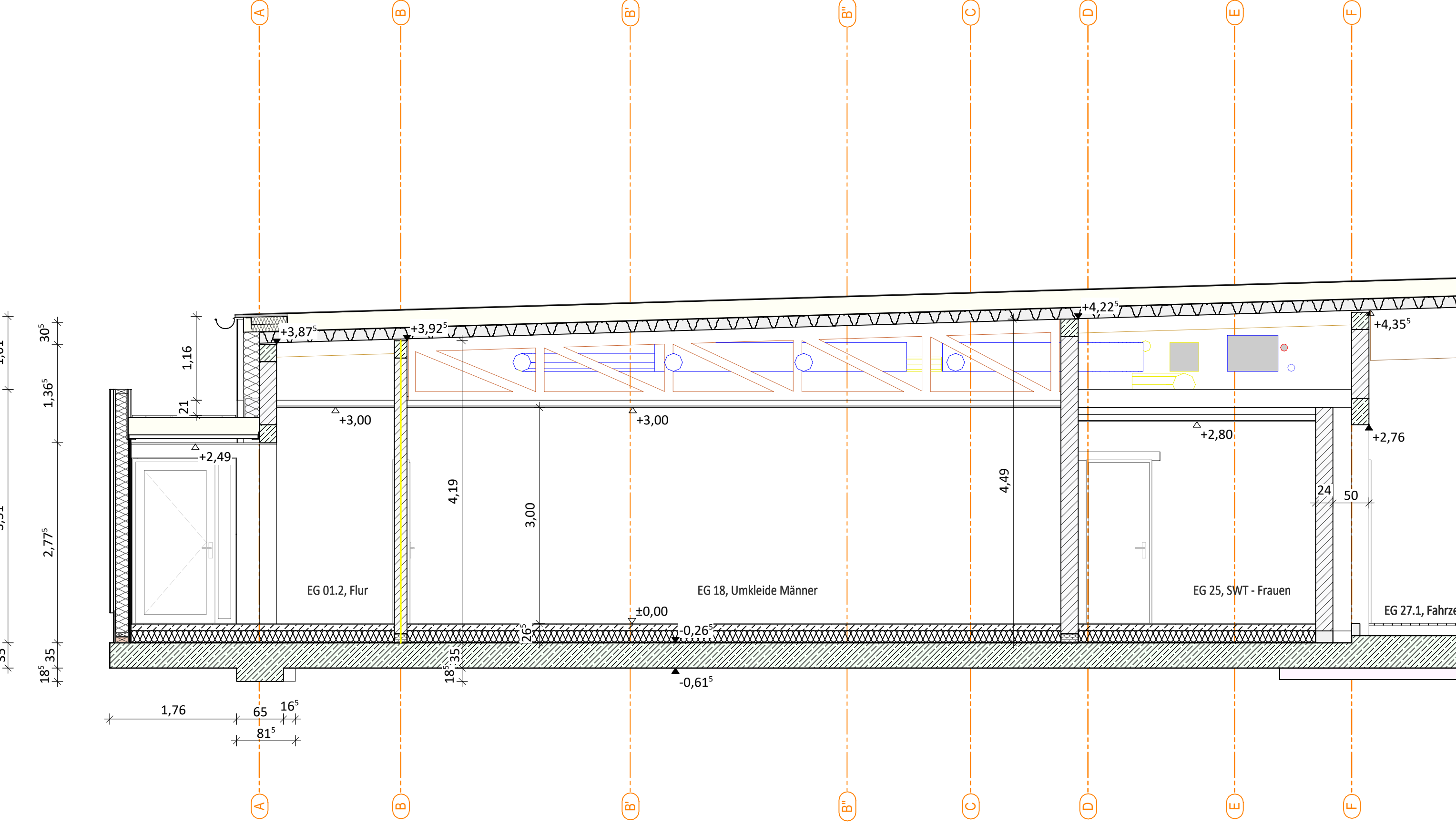
Schnitt F Alarmeingang - Flur - Umkleide H. - Foyer - SWT - Mediennische der Fahrzeughalle
