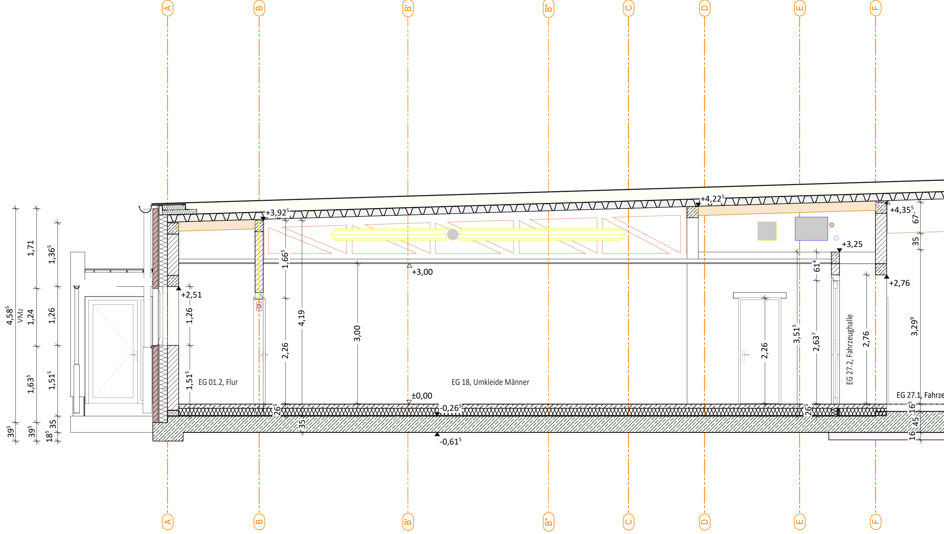
Schnitt E Flur - Umkleide Herren mit Durchgang zur Fahrzeughalle
