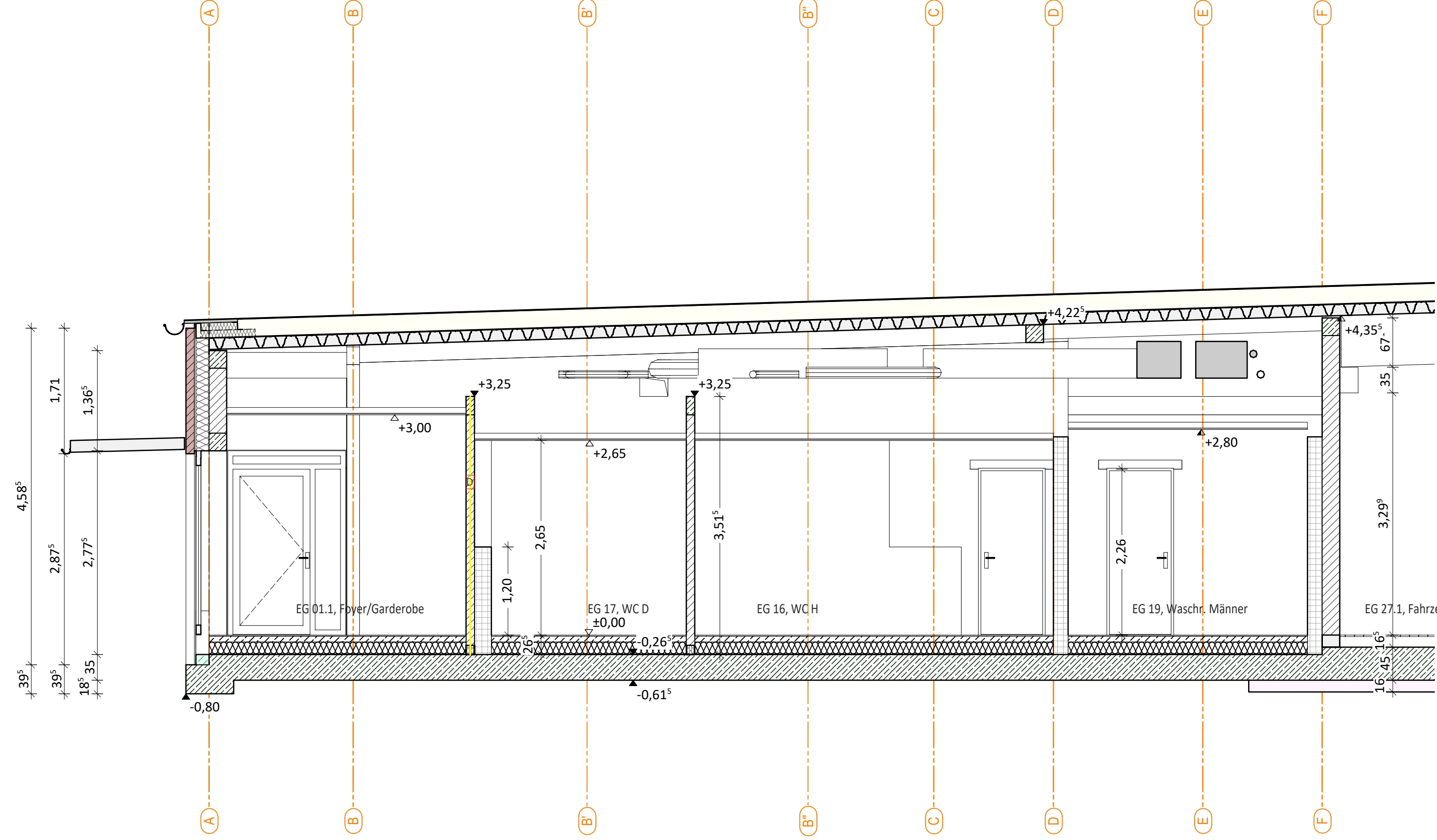
Schnitt D Foyer - WC D - WC Herren - Waschraum Herren
