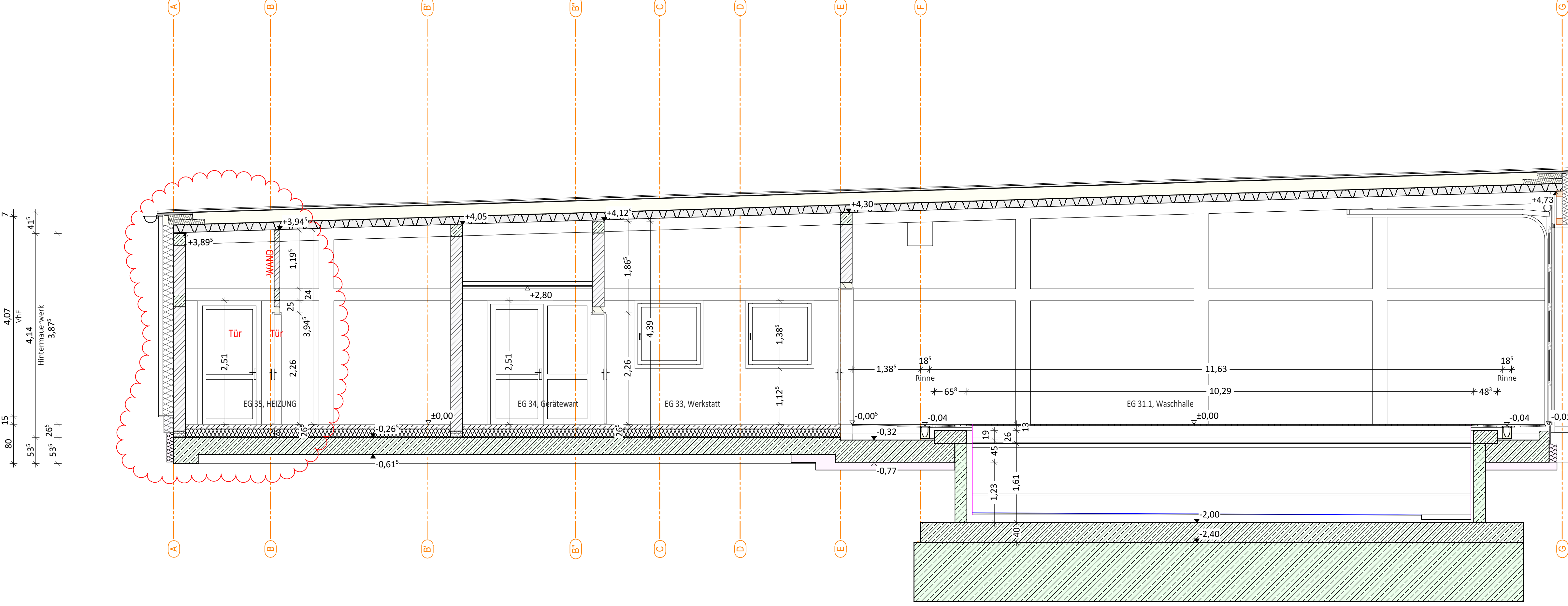
Schnitt H Lager mit eingestelltem Tauschraum - Fahrzeughalle
